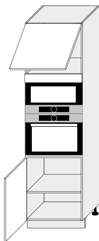
D14/RU/60/207 600/2070/565
