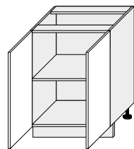
D11/60 600/820/500
