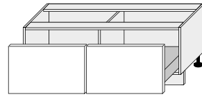
D2E/120 1200/460/500
