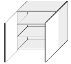
WE/80 800/720/325
