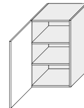
WE/45 450/720/325
