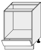
D11K/60 600/820/500
