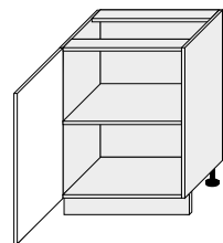
D1D/60 600/820/500
