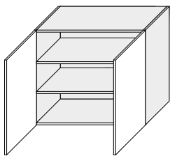
W3/90 900/720/325* 900/720/300**
