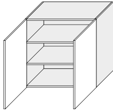
WE/80 800/720/325
