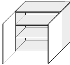
W3/90 900/720/325* 900/720/300**
