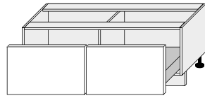
D2M/120 1200/460/500
