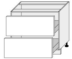
D2E/90 900/820/500
